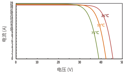
JT665SFk 不同温度下的IV曲线
