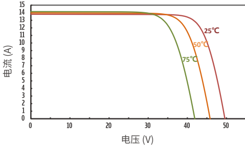
JT540SGh 不同温度下的IV曲线
