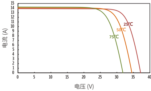
JT405SEh 不同温度下的IV曲线
