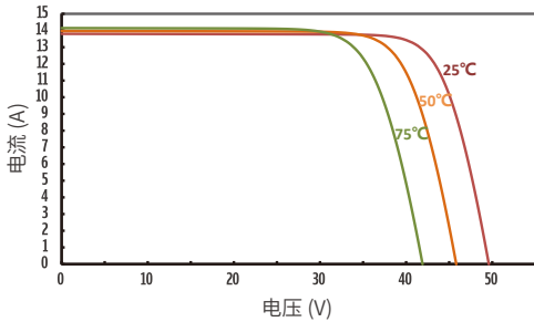
JT540SSh(B) 不同温度下的IV曲线
