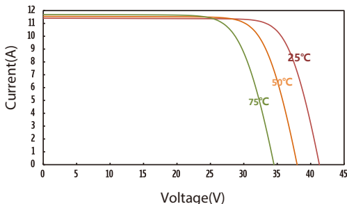
JT370SHh 不同温度下的IV曲线
