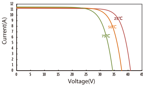
JT360SIh(B) 不同温度下的IV曲线
