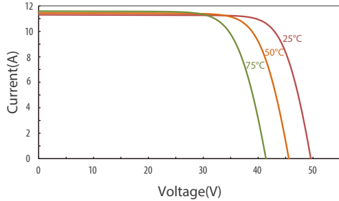
JT440SSh(B) 不同温度下的IV曲线
