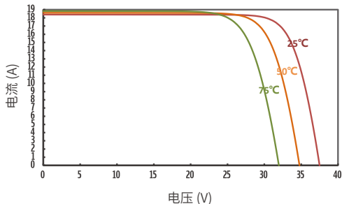
JT550SWk 不同温度下的IV曲线
